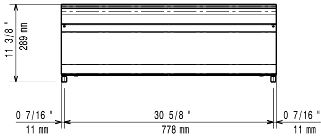
Zij aanzicht
